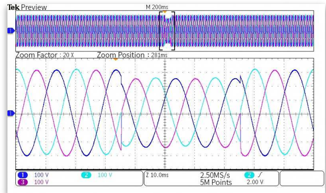
B-C Phase Shift LVRT
