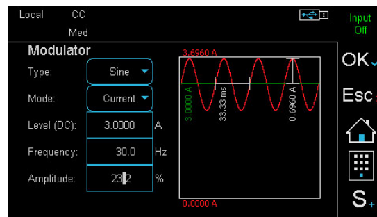
Modulator-Einstellungen
