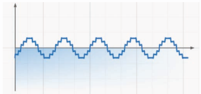
DST26 waveform
