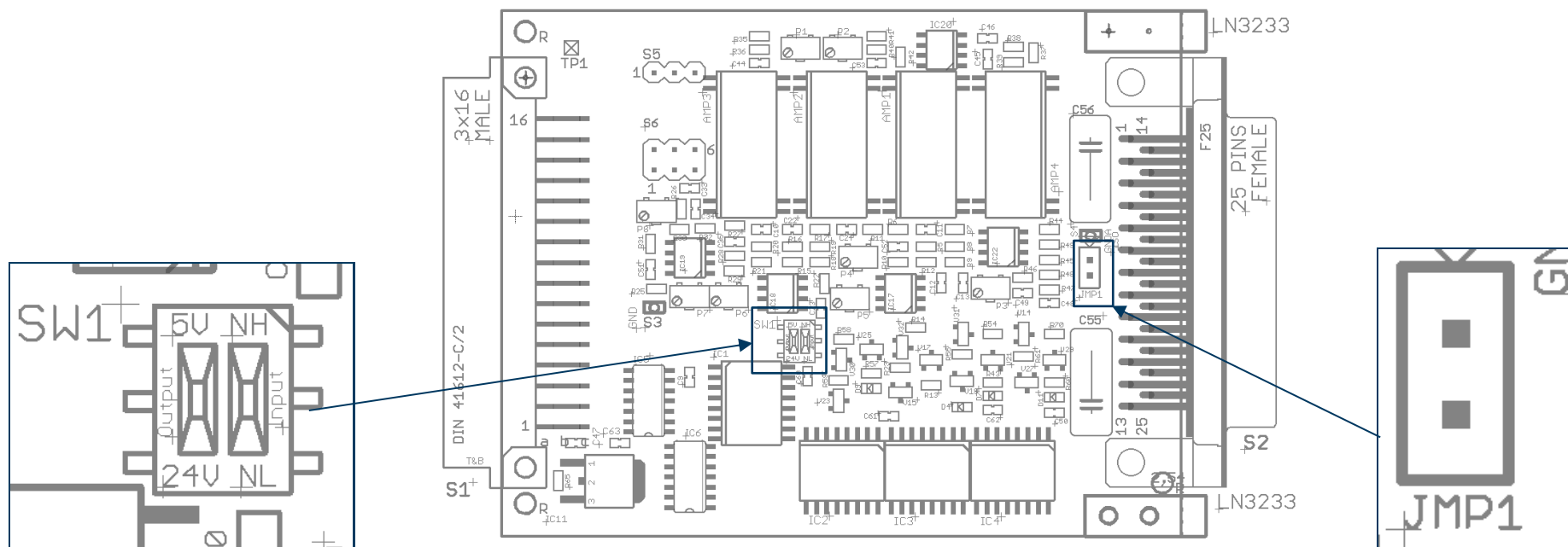
Abbildung 6.2: I/O-Port Board mit SW1 und JMP1
