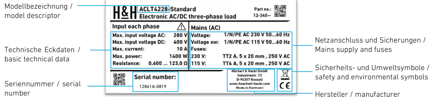
Abbildung 1.1: ACL Typenschild
