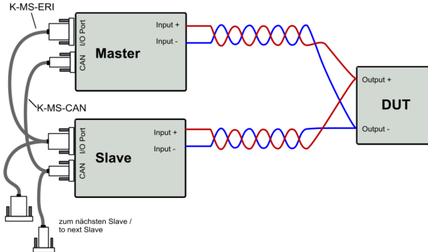
Abbildung 3.5: Verschaltung im Master-Slave-Betrieb Figure 3.5: Wiring in master-slave mode
