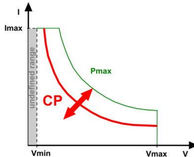
Abbildung 3.2: Leistungsbetrieb (CP)
