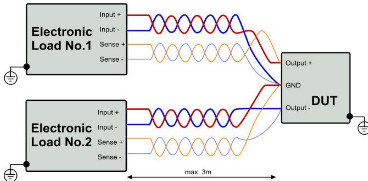
Abbildung 2.3: Anschlussbeispiel für eine bipolare Ausgangsspannung
