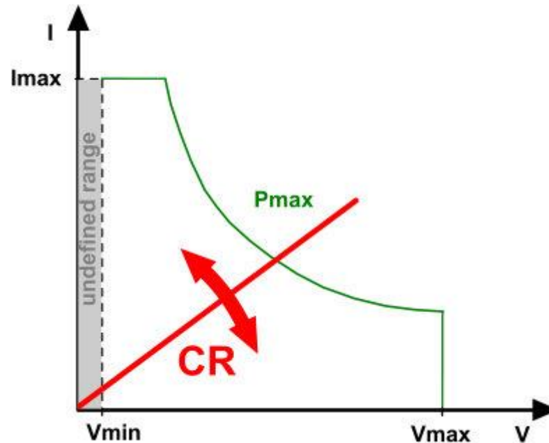
Abbildung 3.3: Widerstandsbetrieb (CR)
