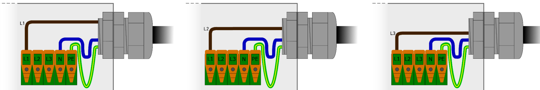
Abbildung 1.3: Symmetrische Verteilung an ein Drehstromnetz mit 3 Geräten ERI36xx
