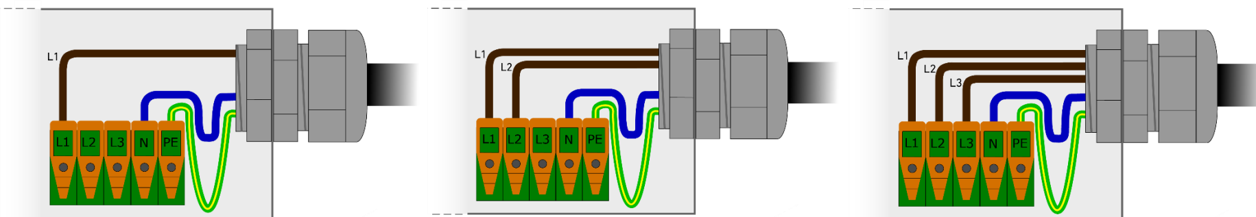
Abbildung 1.2: Verdrahtung des Netzanschlusses bei ERI36xx (l), ERI72xx (m), ERI108xx (r)
