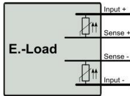
Abbildung 2.4: Interne Beschaltung der Sense-Eingänge Figure 2.4: Internal connection of the sense lines
